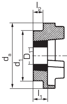
F-Flansch F Flange Bride F Flangia F Brida F
