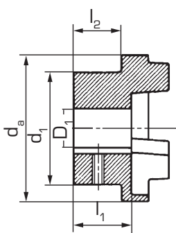
B-Flansch B Flange Bride B Flangia B Brida B
