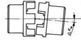
Winkerverlagerung Angular misalignment Défaut d'alignement angulaire Disallineamento angolare Desfase angular
